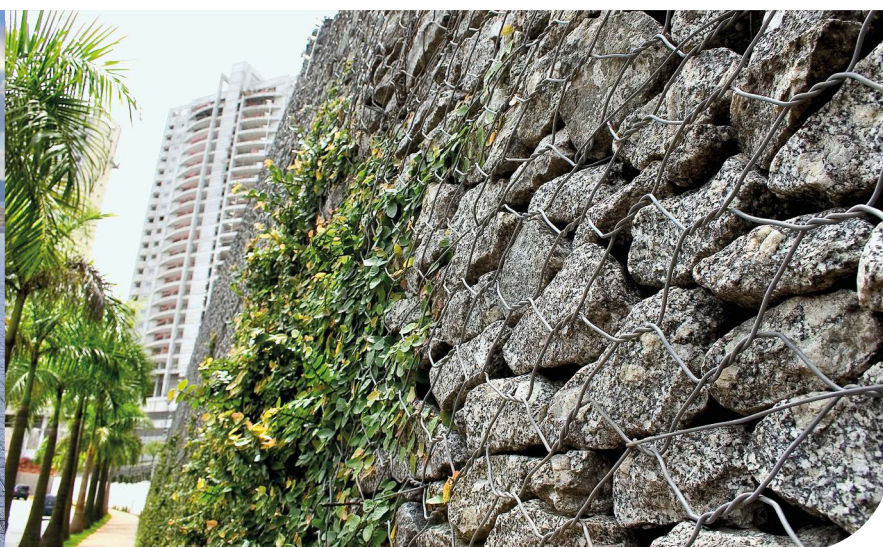
Muro de gravidade com gabiões tecidos
